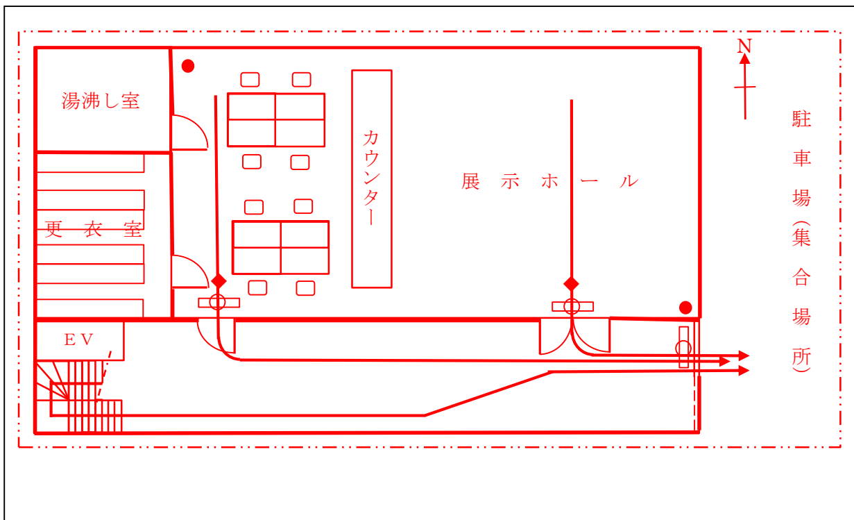
消防用設備等設置位置及び屋外へ通じる避難経路図 (避難経路のみ赤線で記入すること。)
